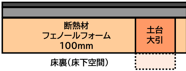
(ア) 土台が 120mm 角でも断熱厚みと揃えて 100mm 厚で計算する
